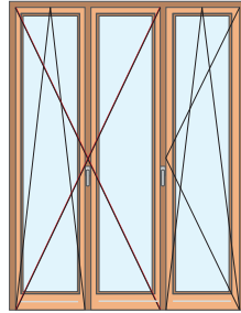
Portafinestra 3 battenti
