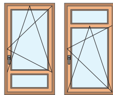
Sottoluce - Sopraluce
